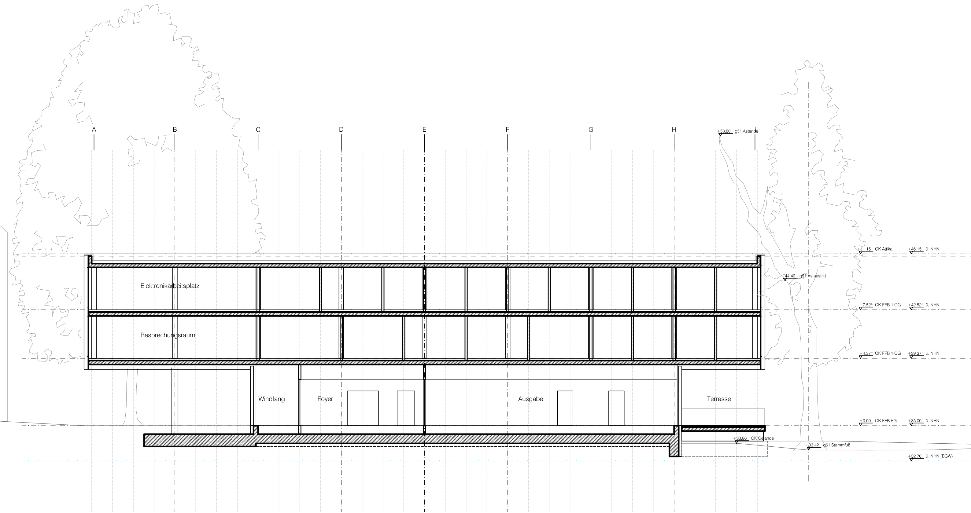
DESY - Neubau SDMC Schnitt A-A, M 1:100, 27.04.2021
