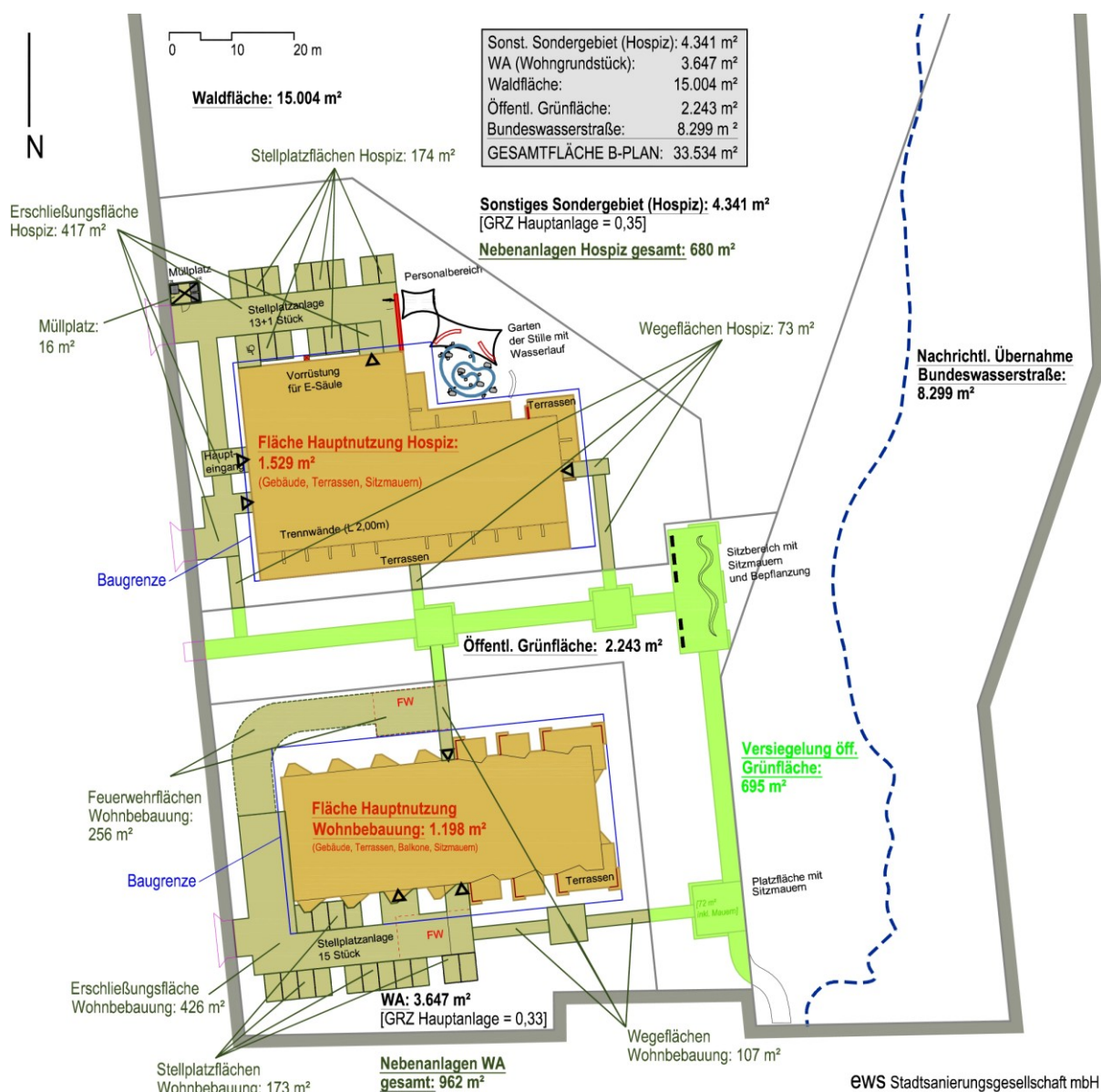
Abb. 25 Flächenversiegelung Plan
