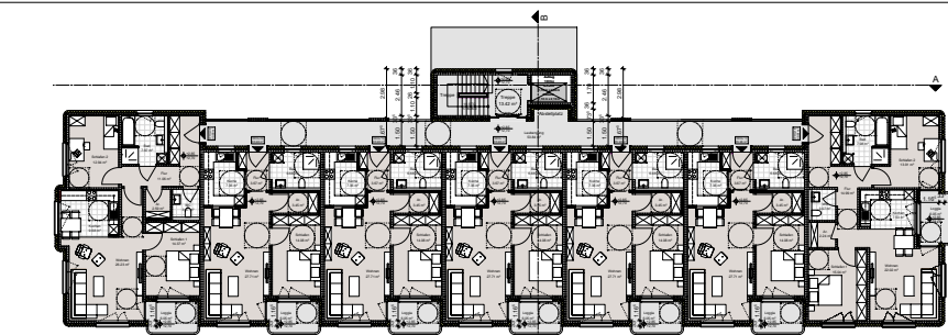
Haus 2 | Grundriss 1.OG - Regelgeschoss M 1:500
